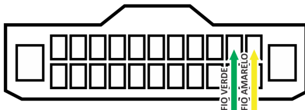
CONECTOR DO RÁDIO ORIGINAL VISTO PELO LADO DOS FIOS
