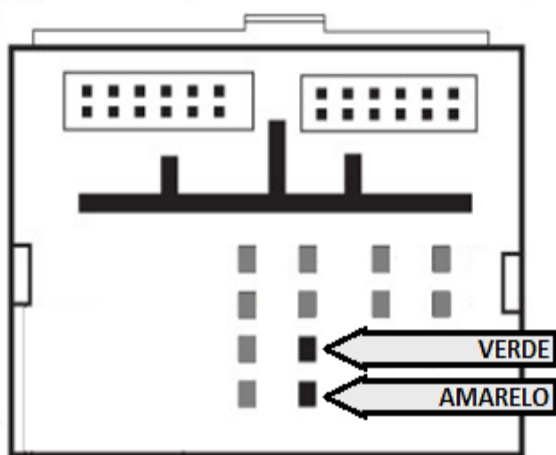
CONECTOR VISTO PELO LADO DOS FIOS.
