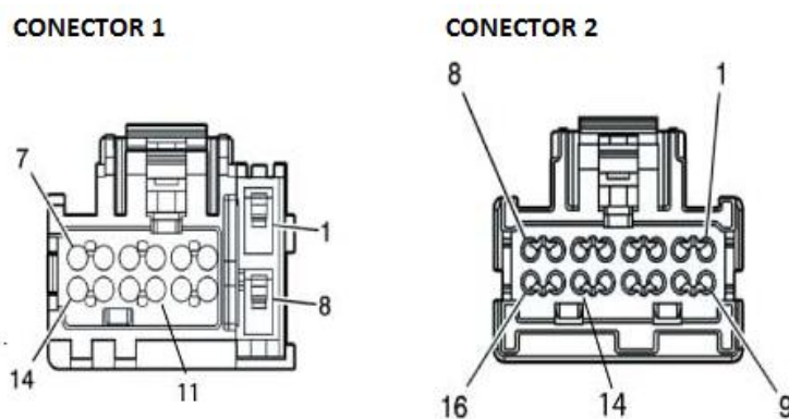
CONECTORES VISTOS DO LADO DOS PINOS, NÃO DOS FIOS.
